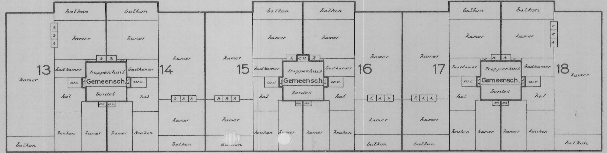
3e Woonlaag 1:200
