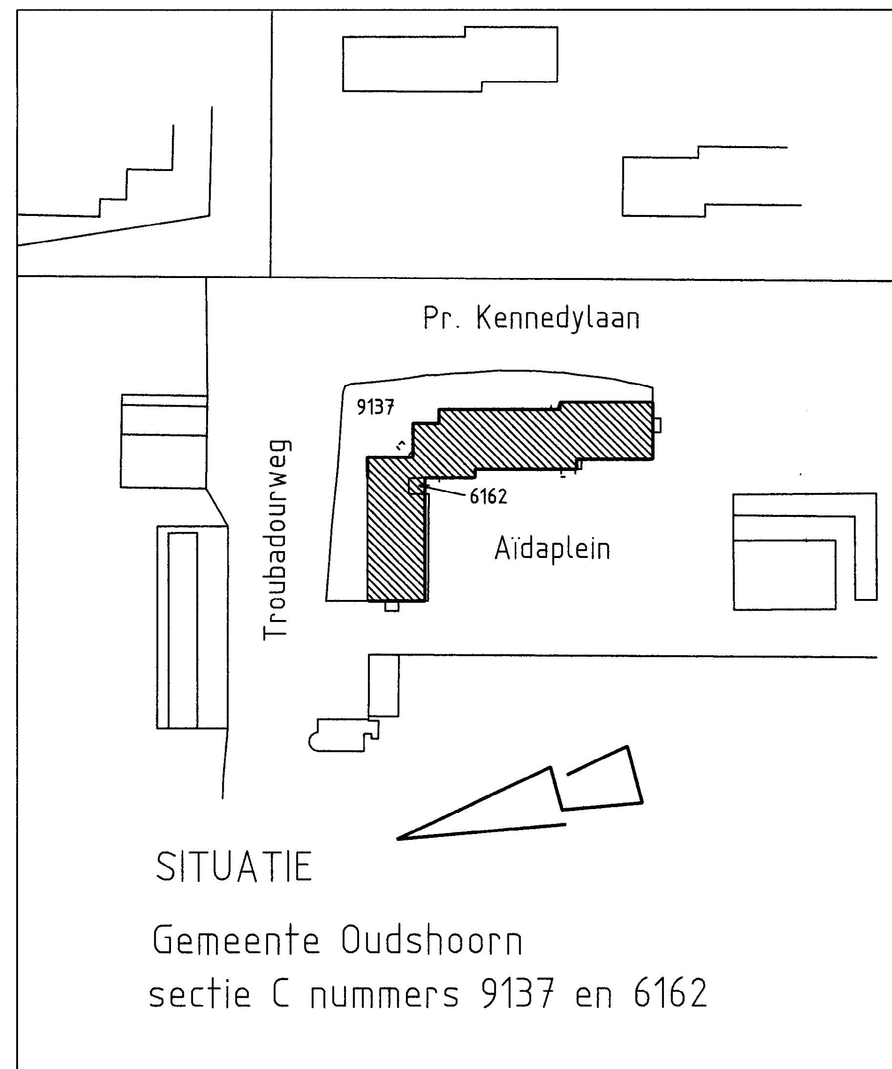
situatie 1:1000
