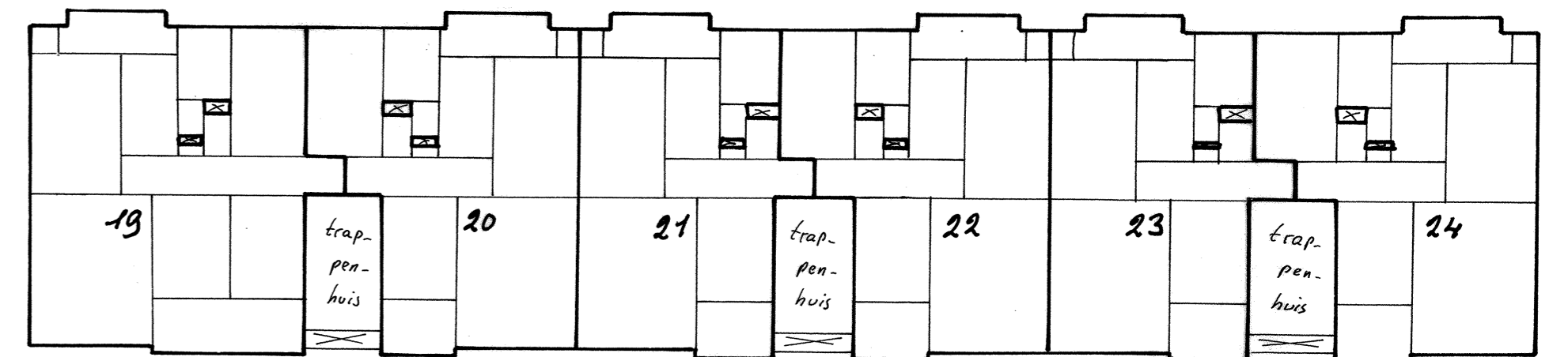
4 e VERDIEPING 1:200
