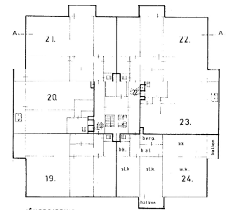
4e VERDIEPING
