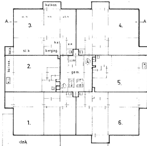
1e VERDIEPING
