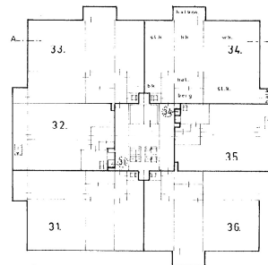
5e VERDIEPING
