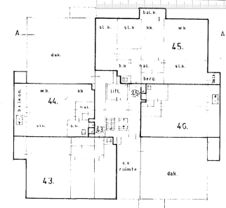
8e VERDIEPING
